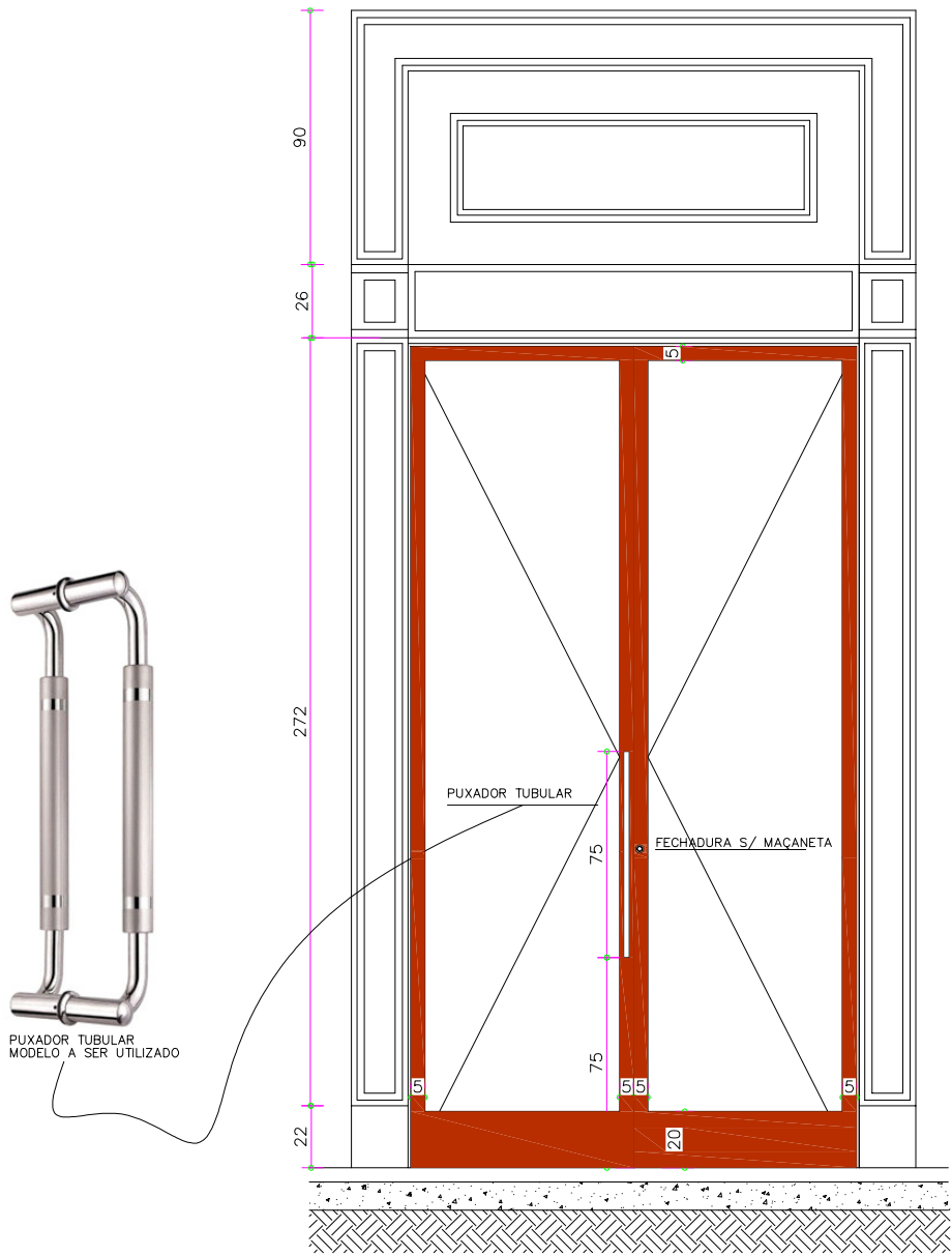
ELEVA[~AO ESCALA: 1/20
